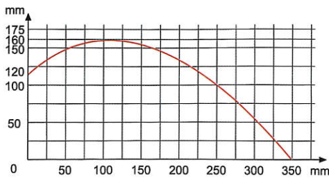
NC-460-3AS 鋸切能力
