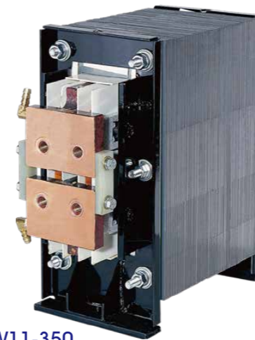
YS-DW11-350 交流熔接變壓器 AC welding transformer 35KVA-50KVA
