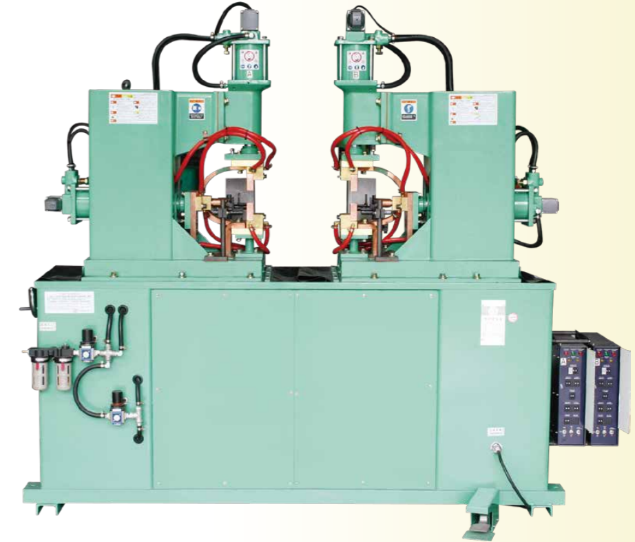
YS-CB100 100KVA H型碰焊熔接機 (2組) Butt Welding Machine, For H shape welds 使用範圍 Application: \phi 1.2~ \phi 2.5
