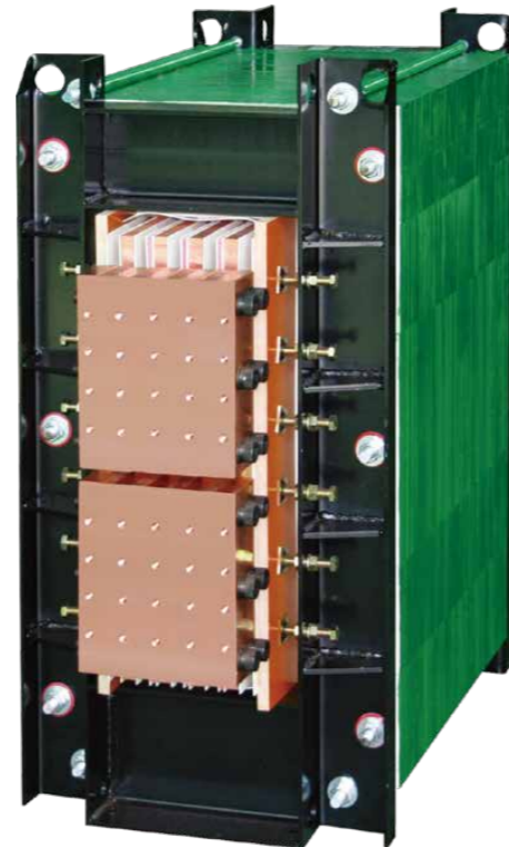
YS-DW21-300 電容式熔接用變壓器 Capacitor Discharge Welding Transformer 30KVA-45KVA
