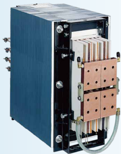
YS-DW21-60 電容式熔接用變壓器 Capacitor Discharge Welding Transformer 6KVA-9KVA
