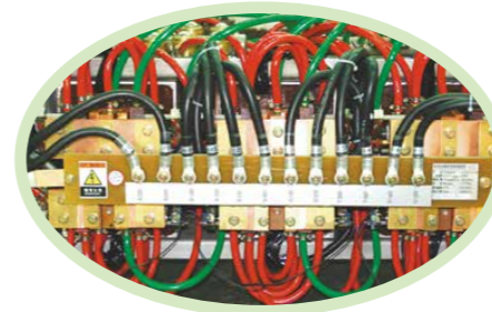
YS-DW52-4500 背式整流型熔接變壓器 DC Welding Transformer(Back-end) 350-750KVA三相入力 Three phase input
