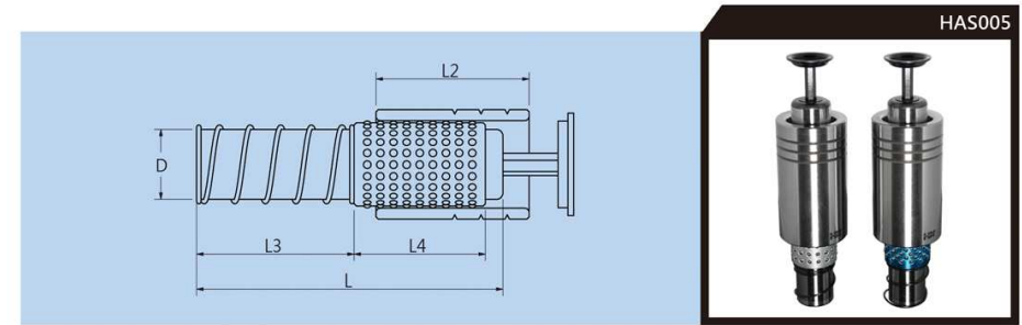
CONSTITUENT PARTS 構成零件
