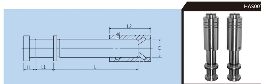
CONSTITUENT PARTS 構成零件
