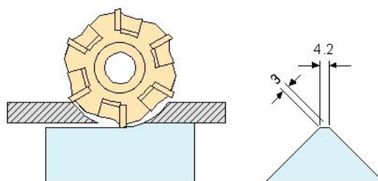
倒角圖示
