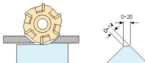
倒角圖示
