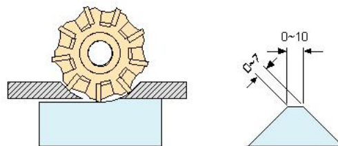
倒角圖示
